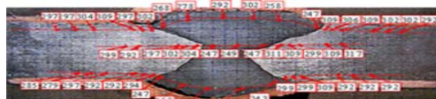
Фиг. 2. Макроструктура на заварено съединение с процес 111
